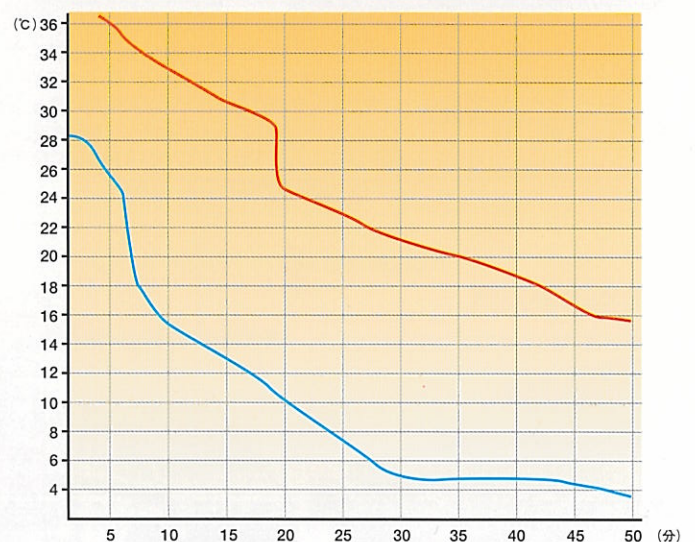
加温停止時室内温度推移
